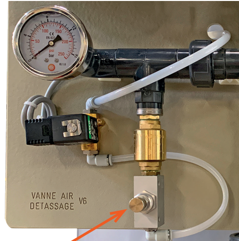
Réglage débit d'air
